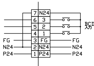
外部接続参考図
